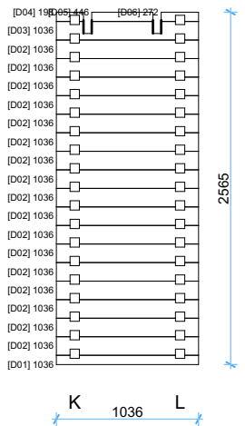
Wall D 1:50
