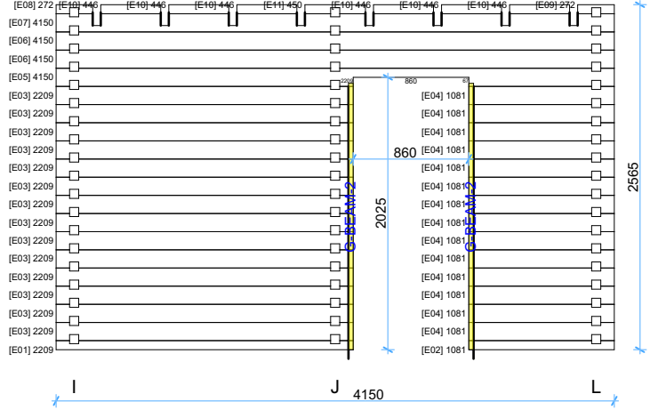
Wall E 1:50
